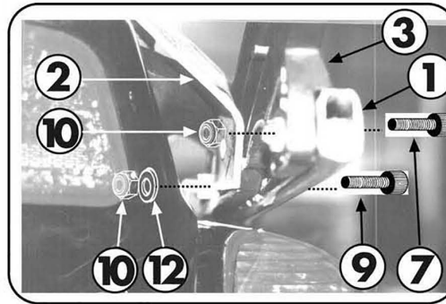
VISTA INTERNA MONTAGGIO SUPPORTO ED ALETTA POSTERIORI ( pz.2 e 3 )
